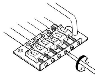
Vis de réglage de l'intonation (pour chaque corde)
