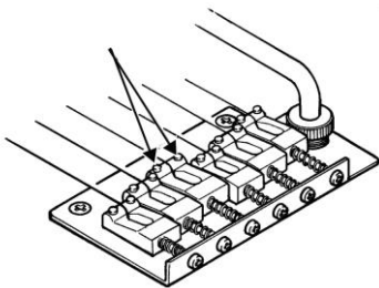
Vis de réglage de la hauteur (pour chaque corde)
